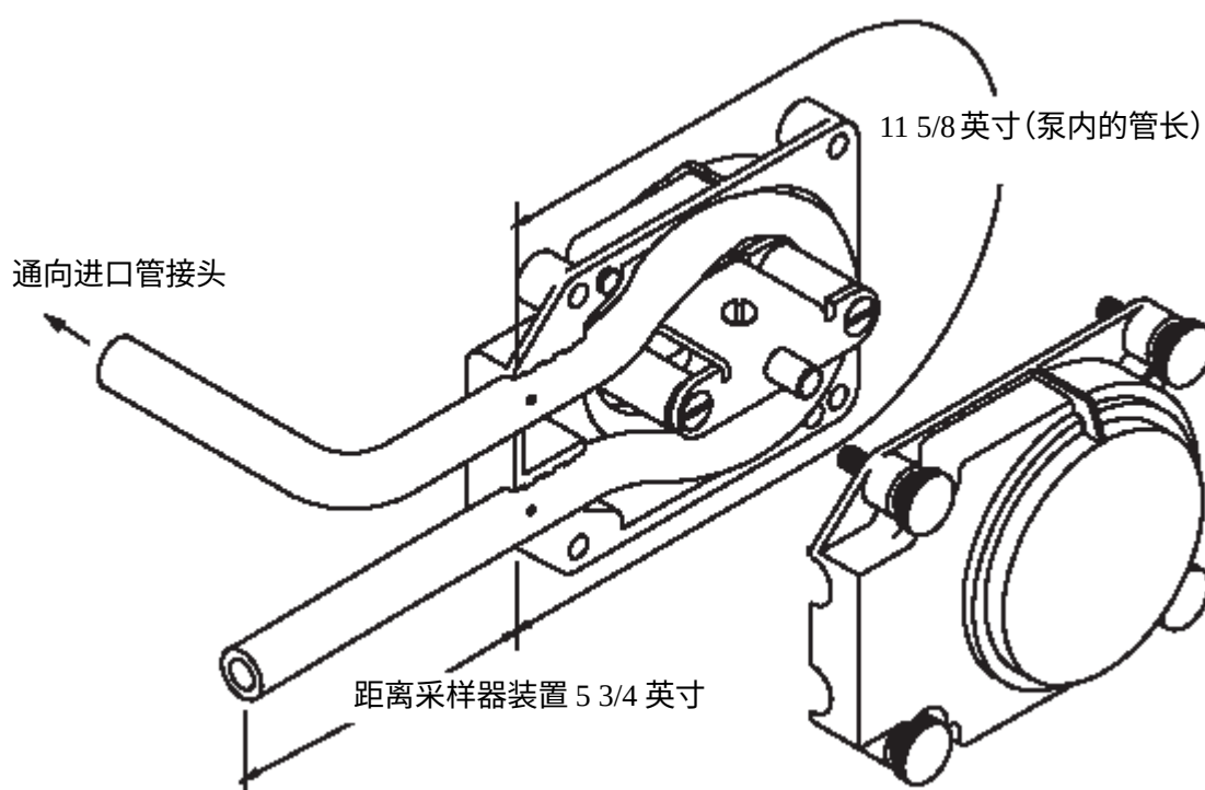
图 32 泵管安装
